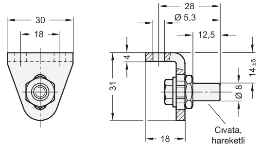
Kilit mandalı braketinin boyutları
